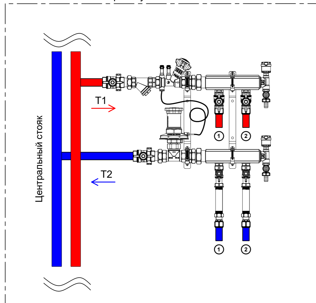
Коллекторный узел этажный GE553-B1
