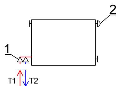
Принципиальная схема с использованием микрометрической компактной группы
