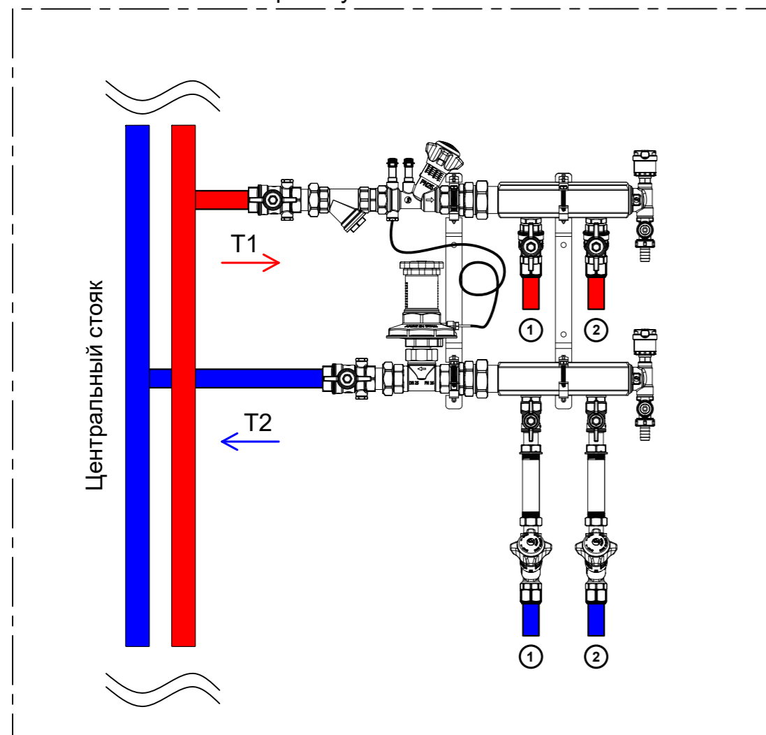
Коллекторный узел этажный GE553-B3
