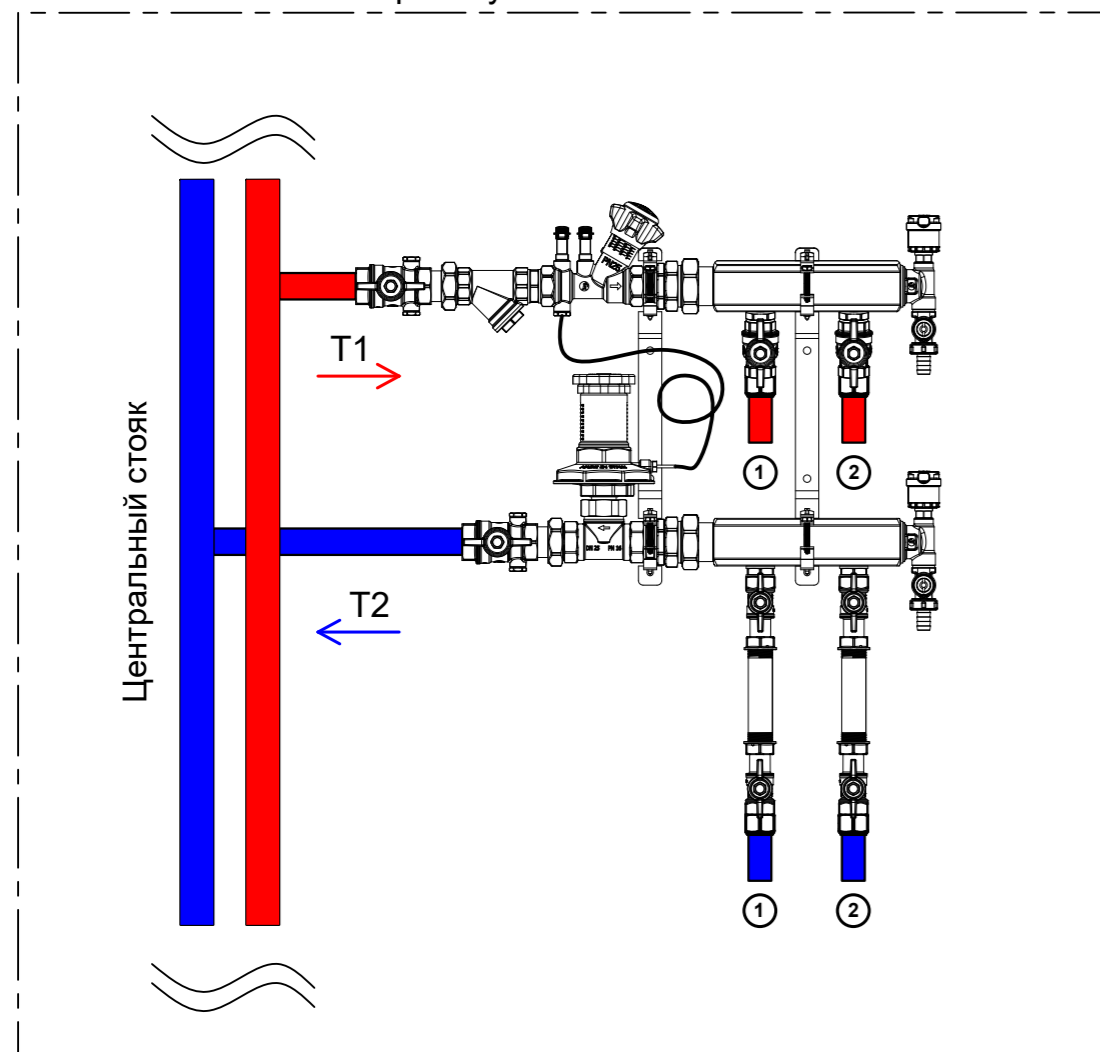
Коллекторный узел этажный GE553-B2
