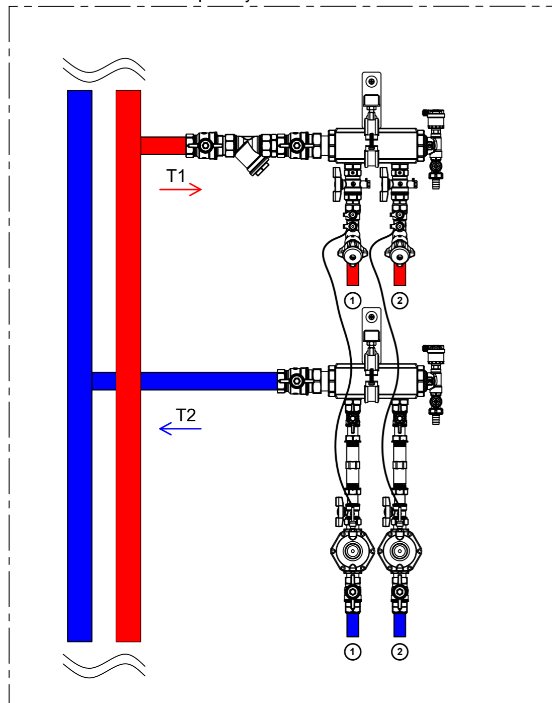
Коллекторный узел этажный GE550-R3
